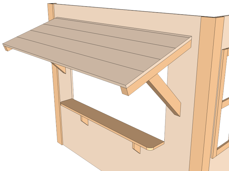
Stříška nad pultíkem (detail bez lišt)
